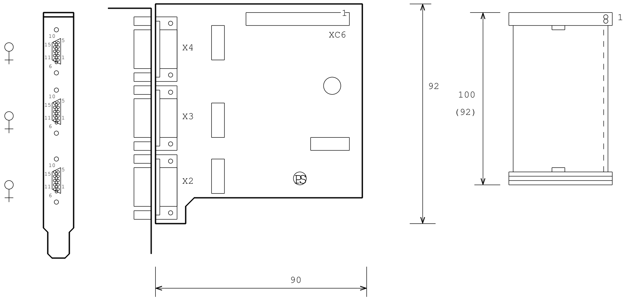
NACRTEK JEDNOTKY SU05 (druha cast desky)
