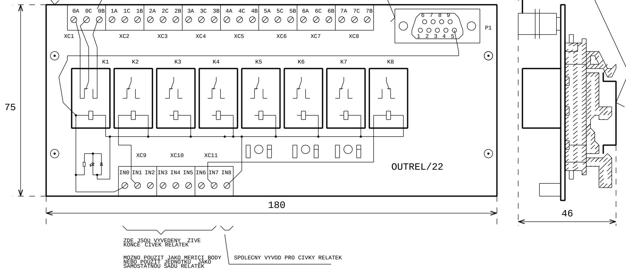
ROZMEROVÝ NACRTEK JEDNOTKY OUT06
