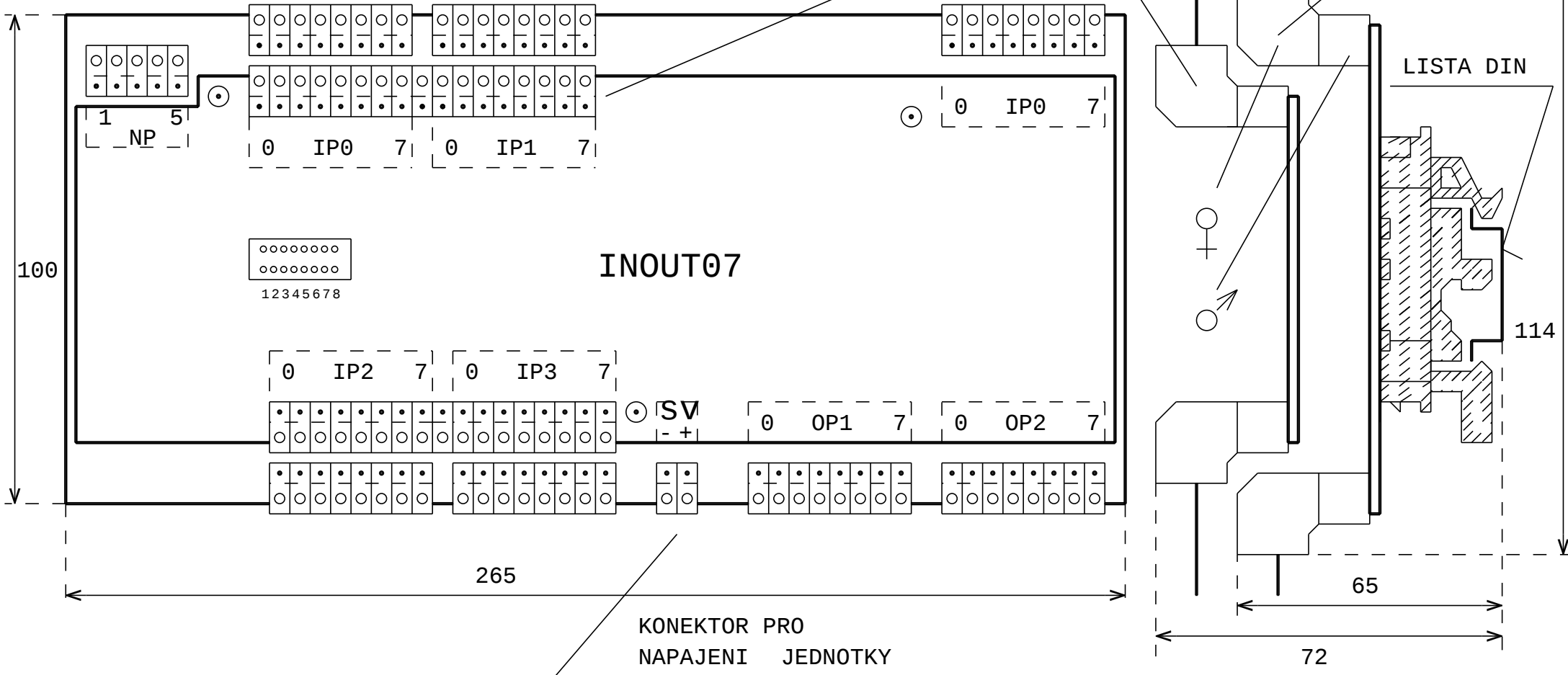
ROZMEROVY NACRTEK JEDNOTKY INOUR07
